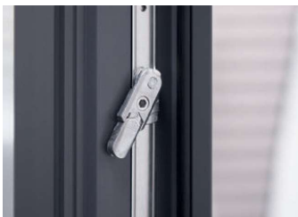
Zasuwnica z blokadą obrotu klamki i podnośnikiem skrzydła
