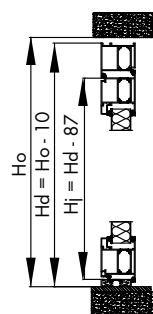
Rys. 70. Montaż w otworze - przekrój pionowy - drzwi jednoskrzydłowe - system MB70.
